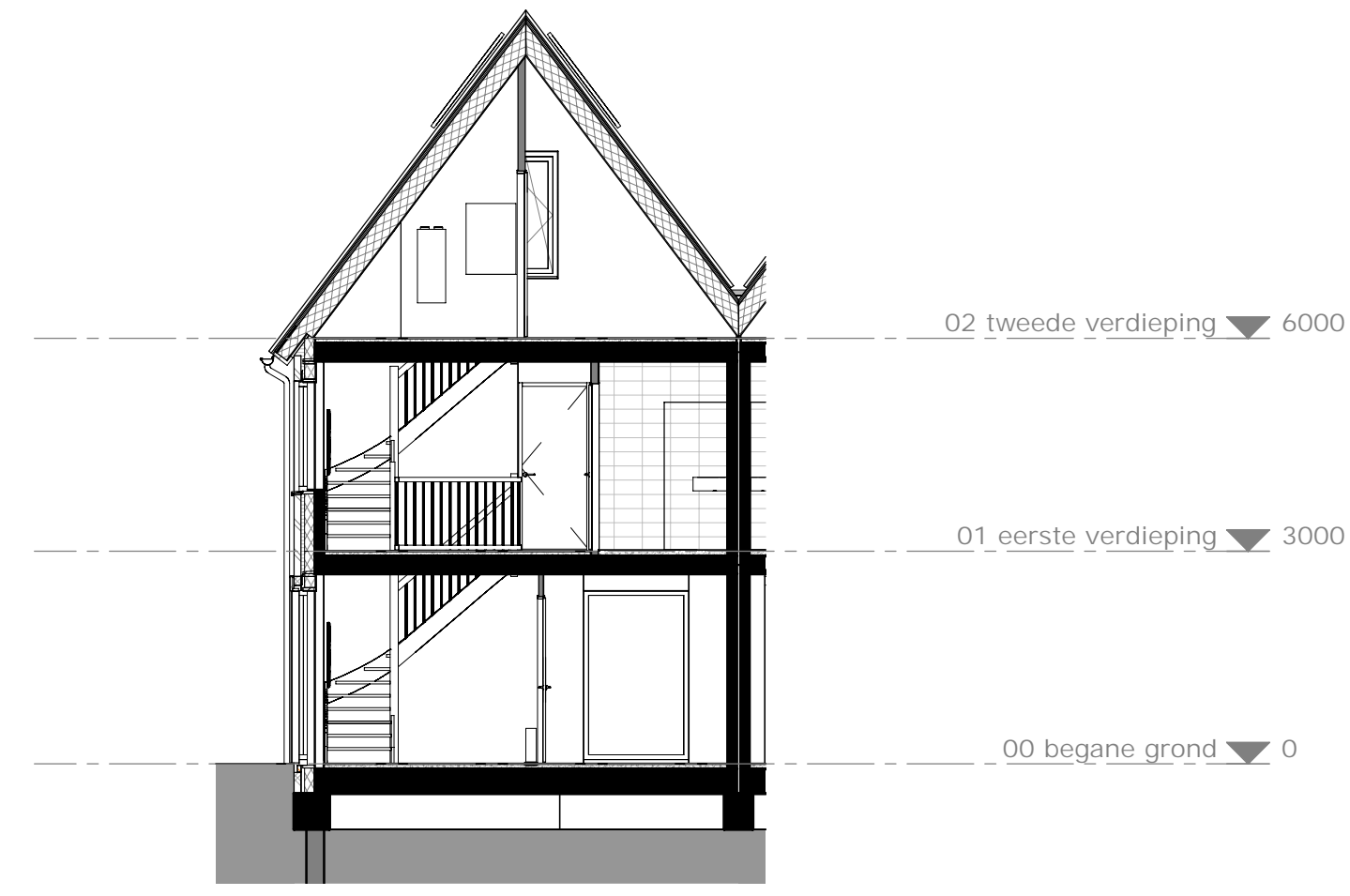
doorsnede 2 schaal 1:100
