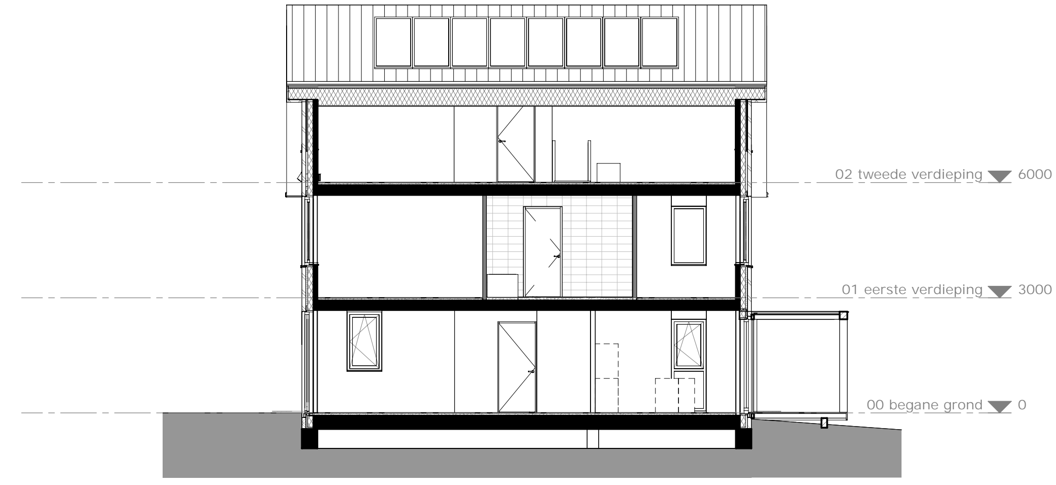
doorsnede 1 schaal 1:100
